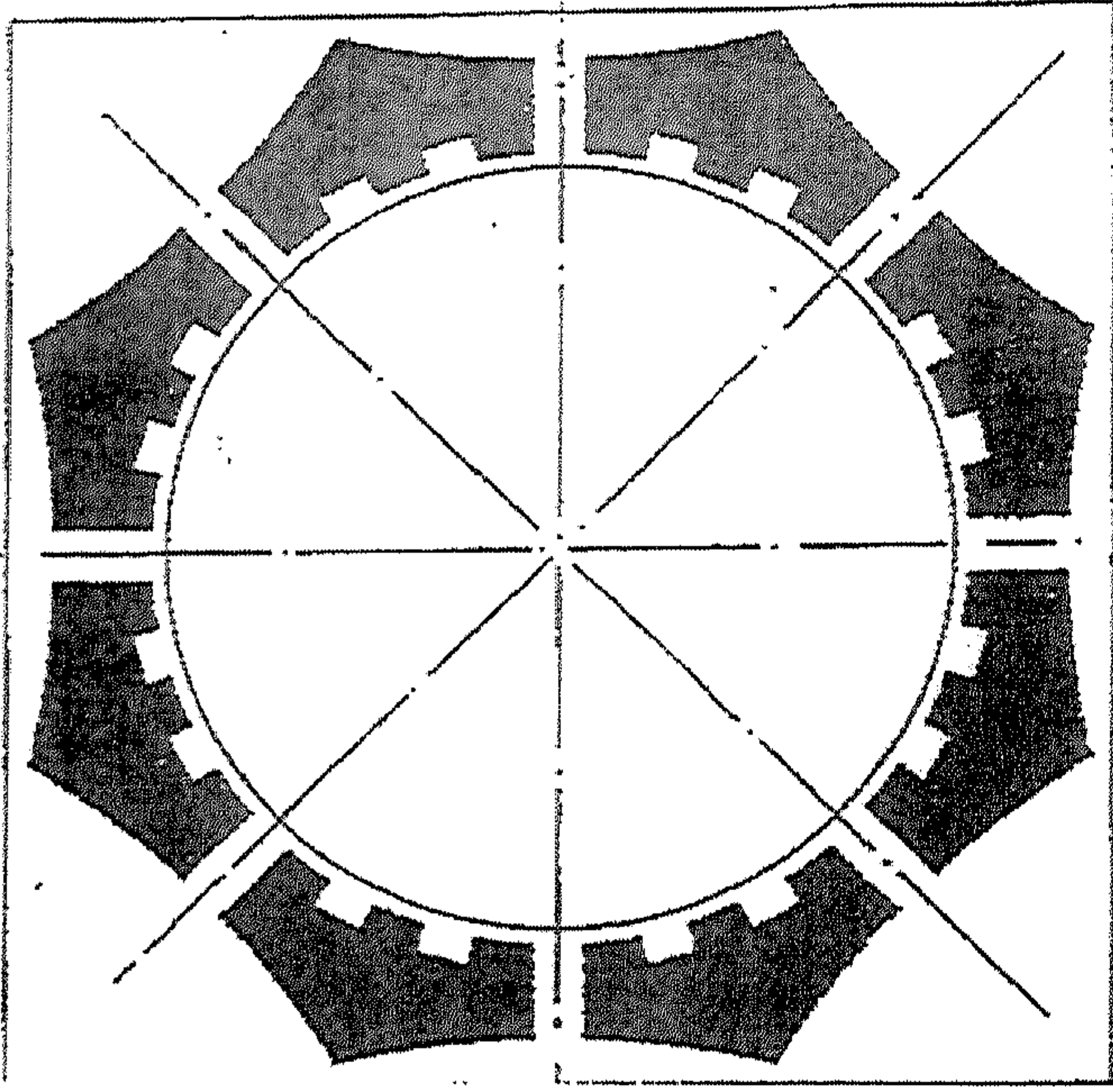
(شكل رقم ٥٣) رسم تخطيطي لقبة المحراب بجامع القبروان عن ليزين.
